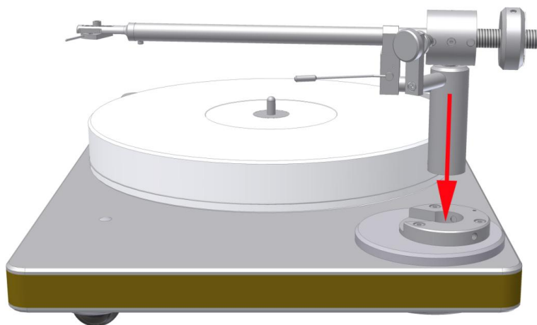
Bild 2: Befestigung des Tonarms an der Rundbasis
